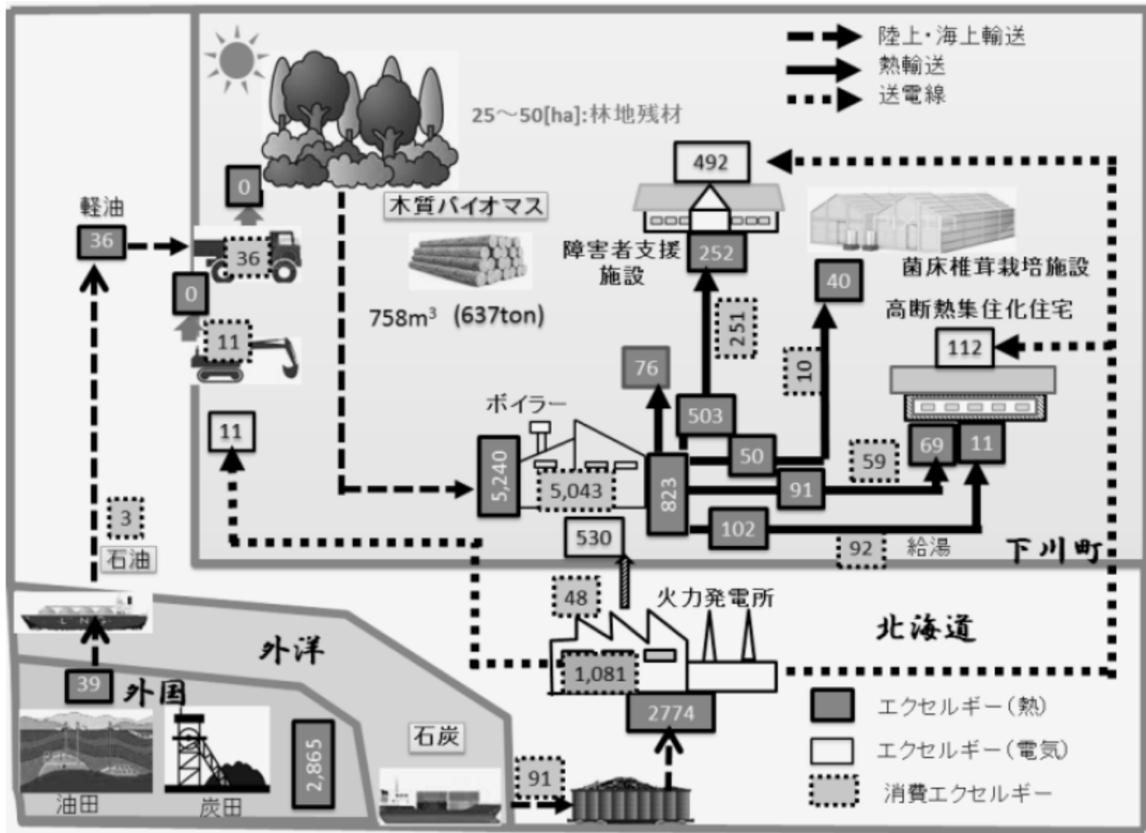
出典：山崎 慶太(竹中工務店)・斉藤 雅也(札幌市立大学)・宿谷 昌則(東京都市大学)：林業から住宅・バイオマスを利用した地域熱供給の事例紹介、日本建築学会 環境工学委員会 第45回熱シンポジウム予稿集, pp.131-138, 2015.11.
